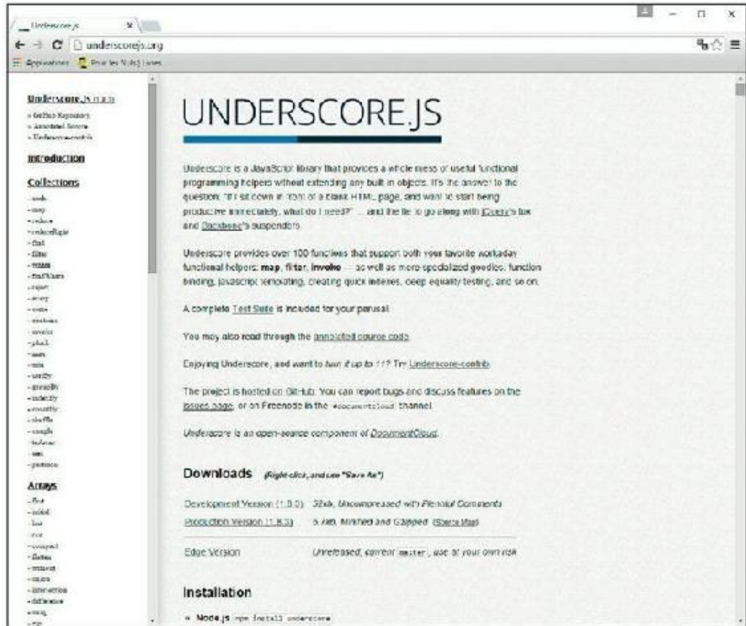
FIGURE 19.7 : http://underscorejs.com .
